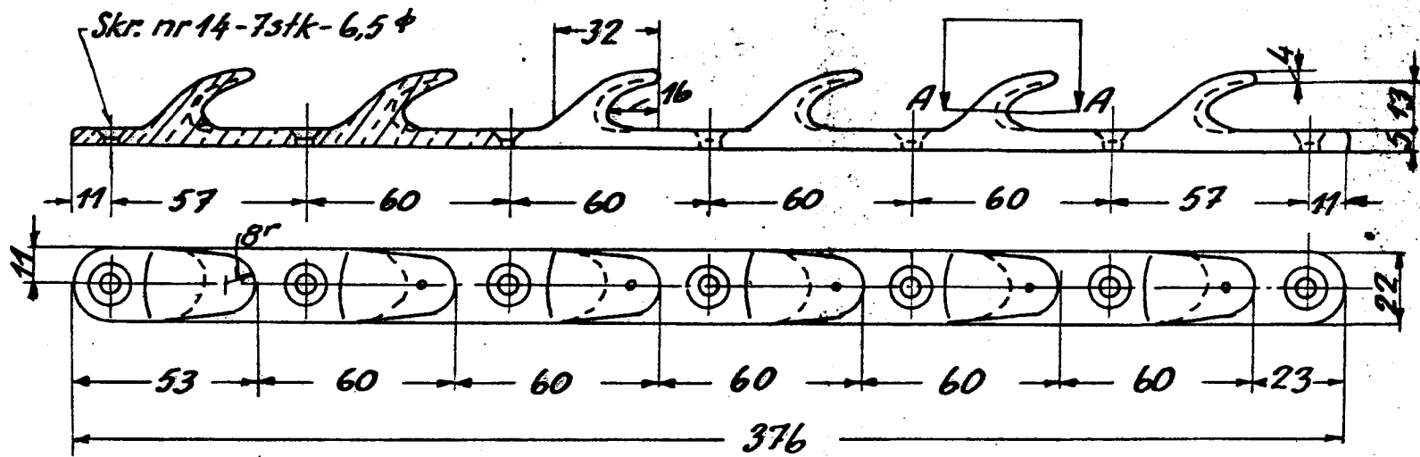
Hakeskinne \phi 13
