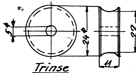
Skråblokk for spinakerskjöt \phi -15
